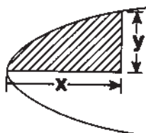
Parabola
