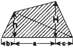
Trapezium
