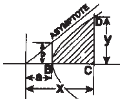
Hyperbola
